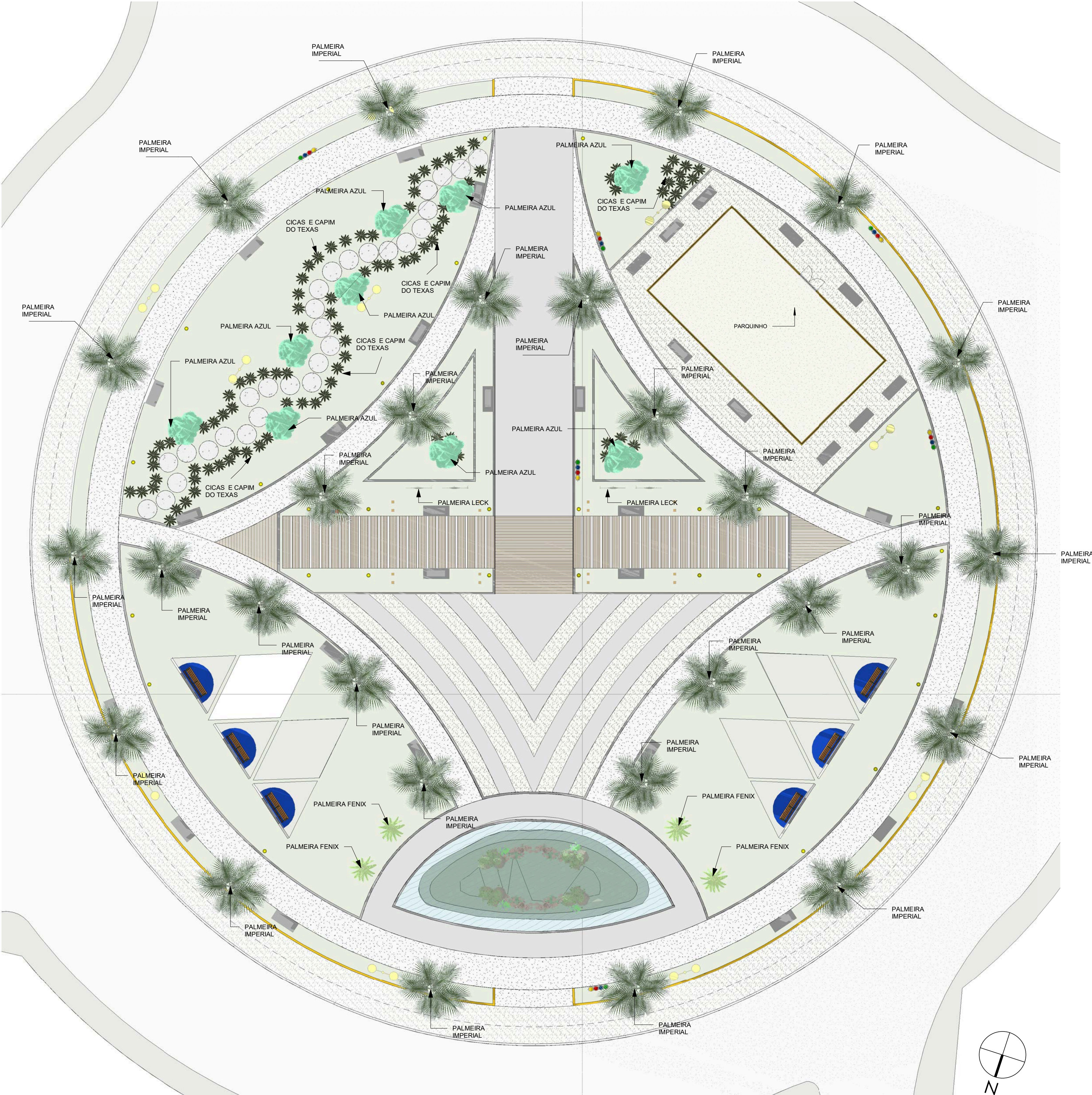
1 PLANTA DE PAISAGISMO ESCALA - 1 : 200
