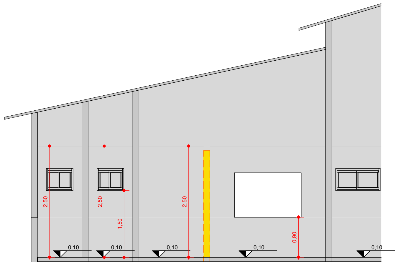
5 CORTE TRANSVERSAL- DEMOLIR PAREDE ESCALA - 1 : 50
