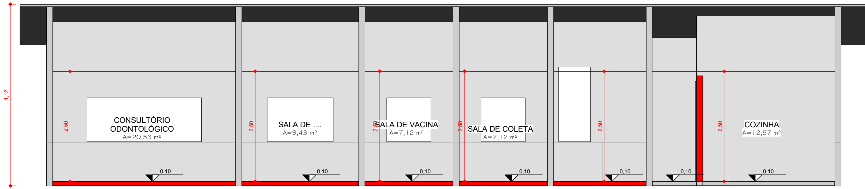
4 CORTE 1 - CONSTRUIR ESCALA - 1 : 50
