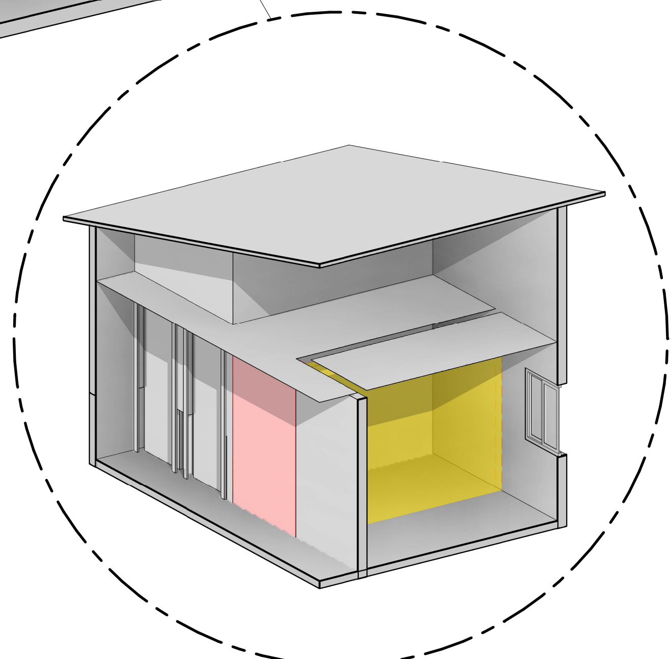
6 PESPECTIVA DEMOLIR/ CONSTRUIR PAREDES ESCALA -
